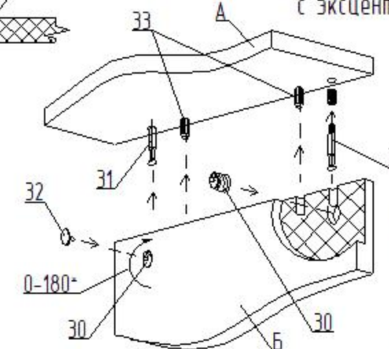
Пример монтажа стыкуемых панелей с эксцентриковыми стяжками и шкантами
