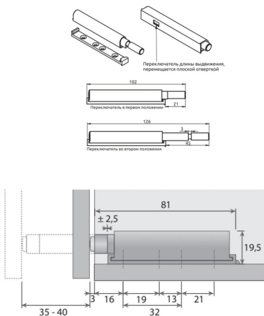
Схема установки и регулировки толкателя!
